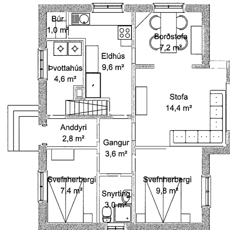
Jarðhæð; 1:100
