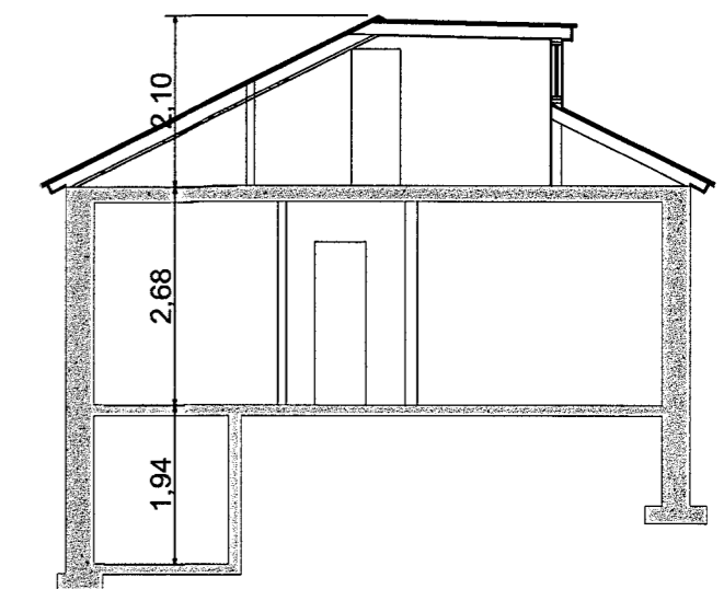
Snið 1-1; 1:100
