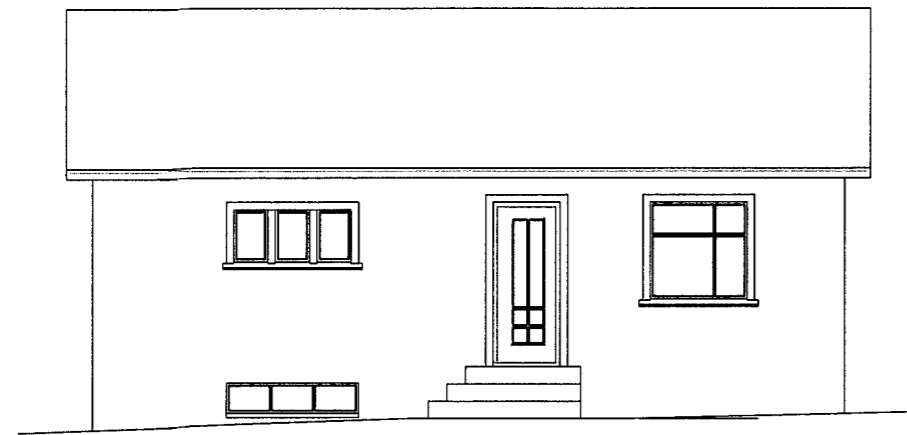
Austurhlið; 1:100
