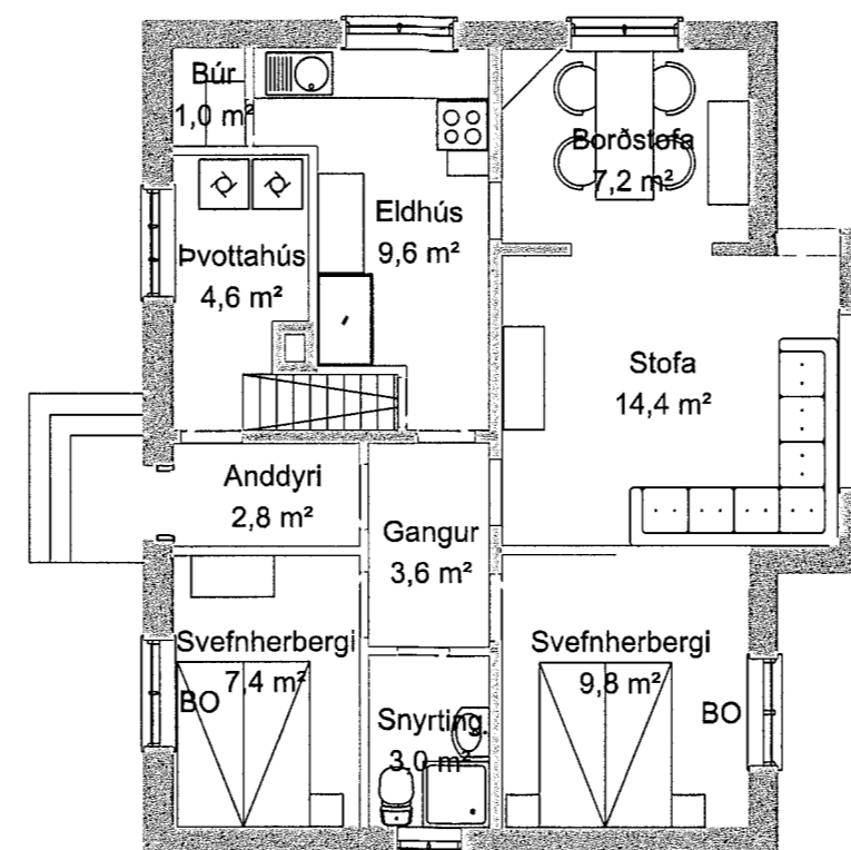
Jarðhæð; 1:100
