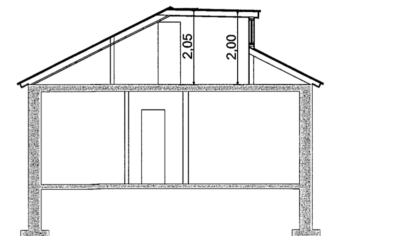
Snið 1-1; 1:100
