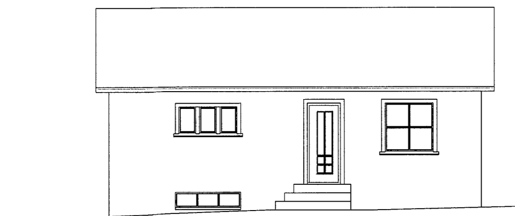
Austurhlið; 1:100
