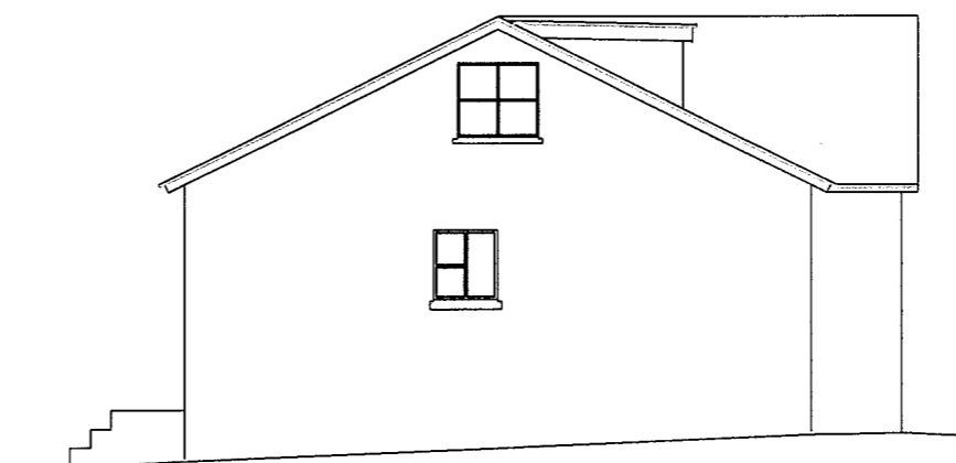
Norðurhlið; 1:100
