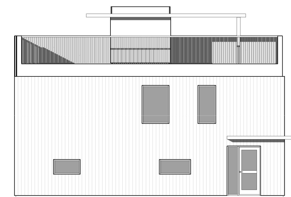
Vestur mkv: 1 : 100
