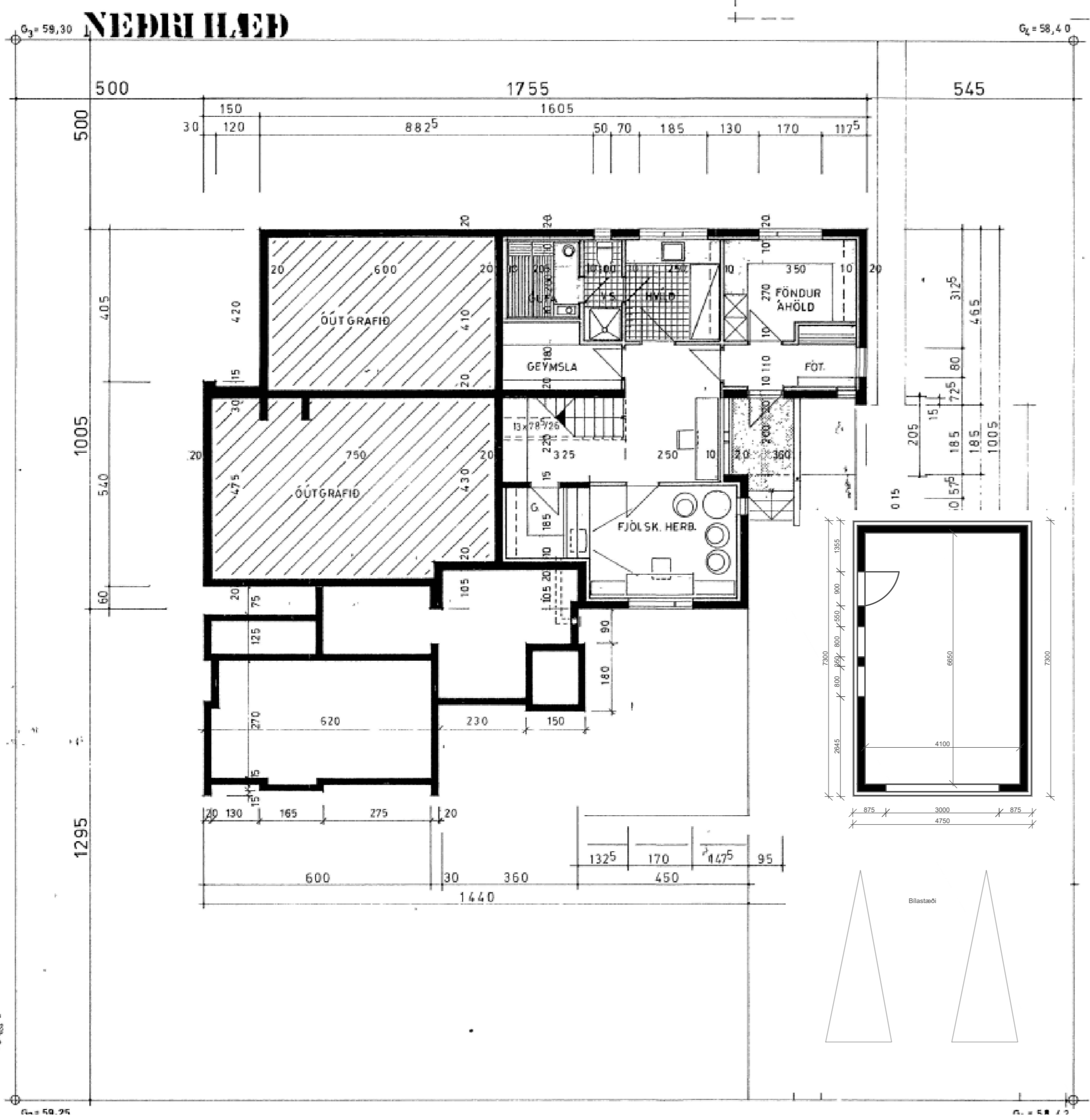
Grunnmynd neðri hæð M 1:100
