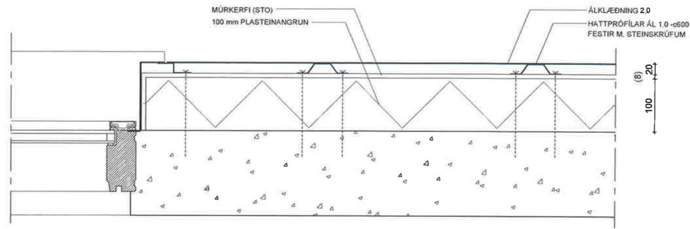
DEILI 1 LÁRÉTT SNID Í VEGG
