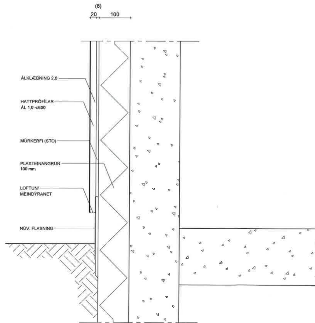
DEILI 2 LÓÐRÉTT SNID Í VEGG
