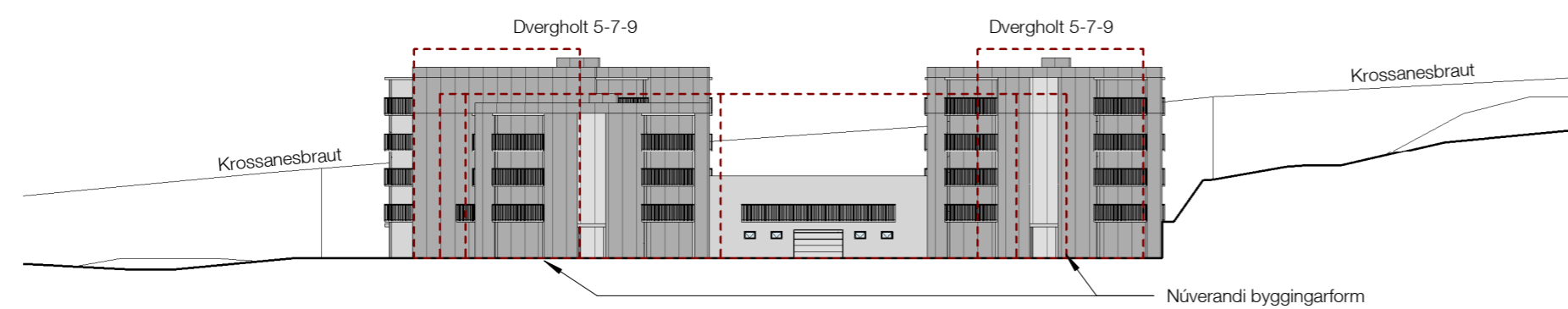
Snið A-A 1:500
