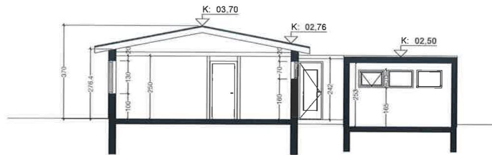
Snið A-A 1:100
