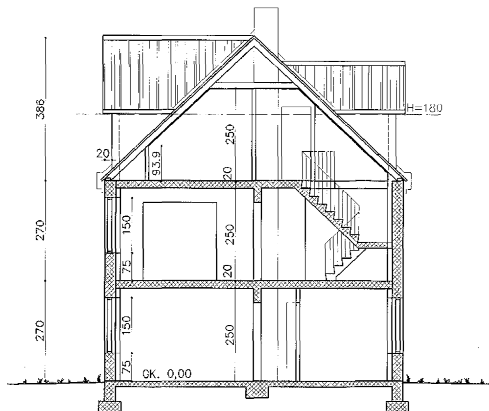
SNID A-A 1:100
