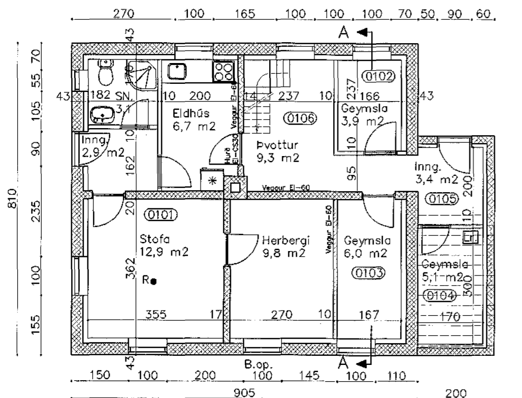
KJALLARI 1:100
