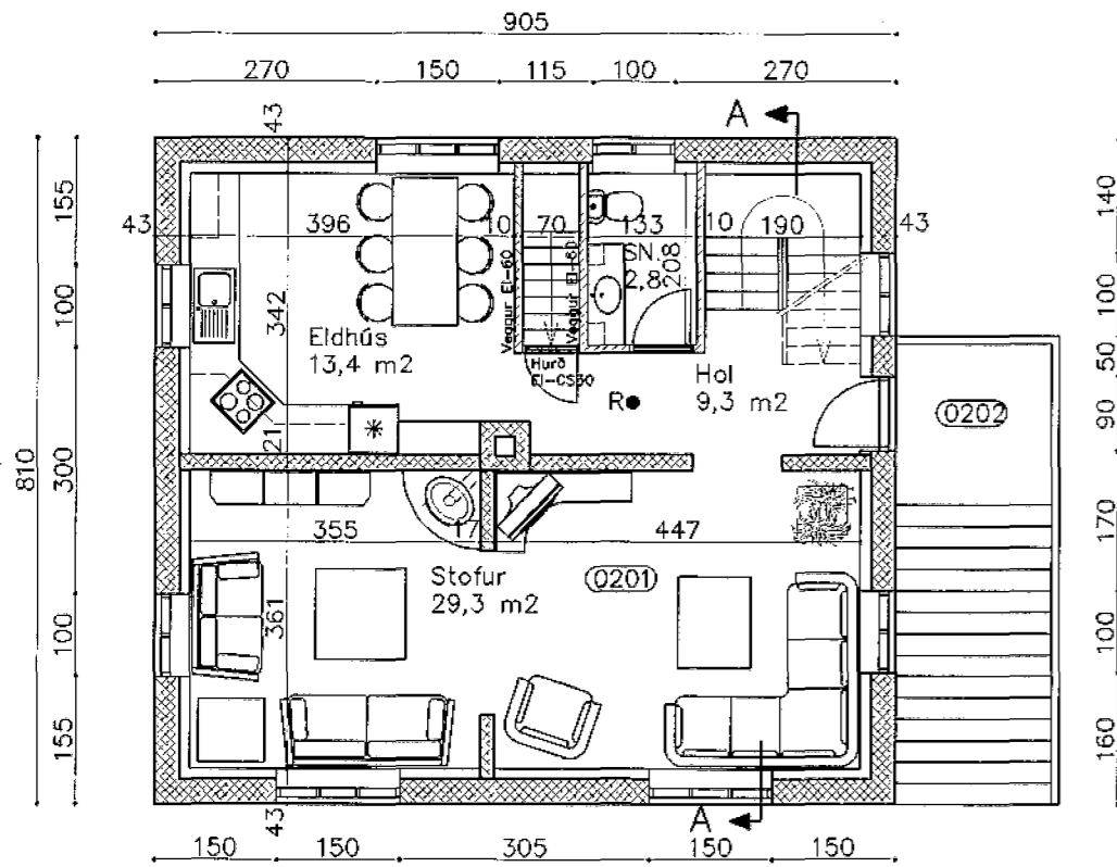
2.HÆÐ 1:100
