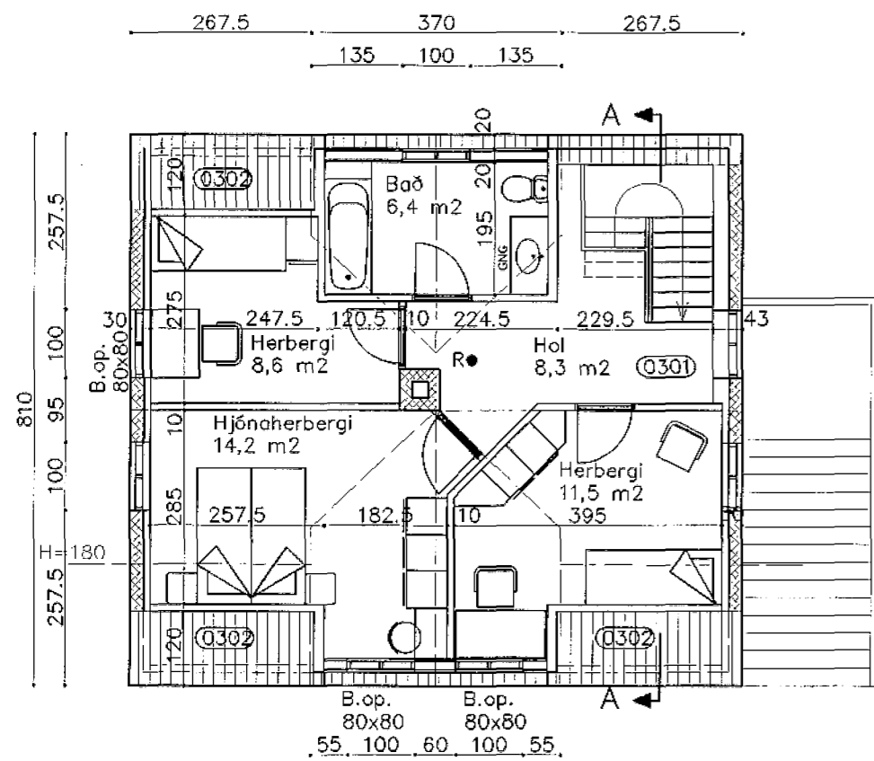
3.HÆÐ 1:100
