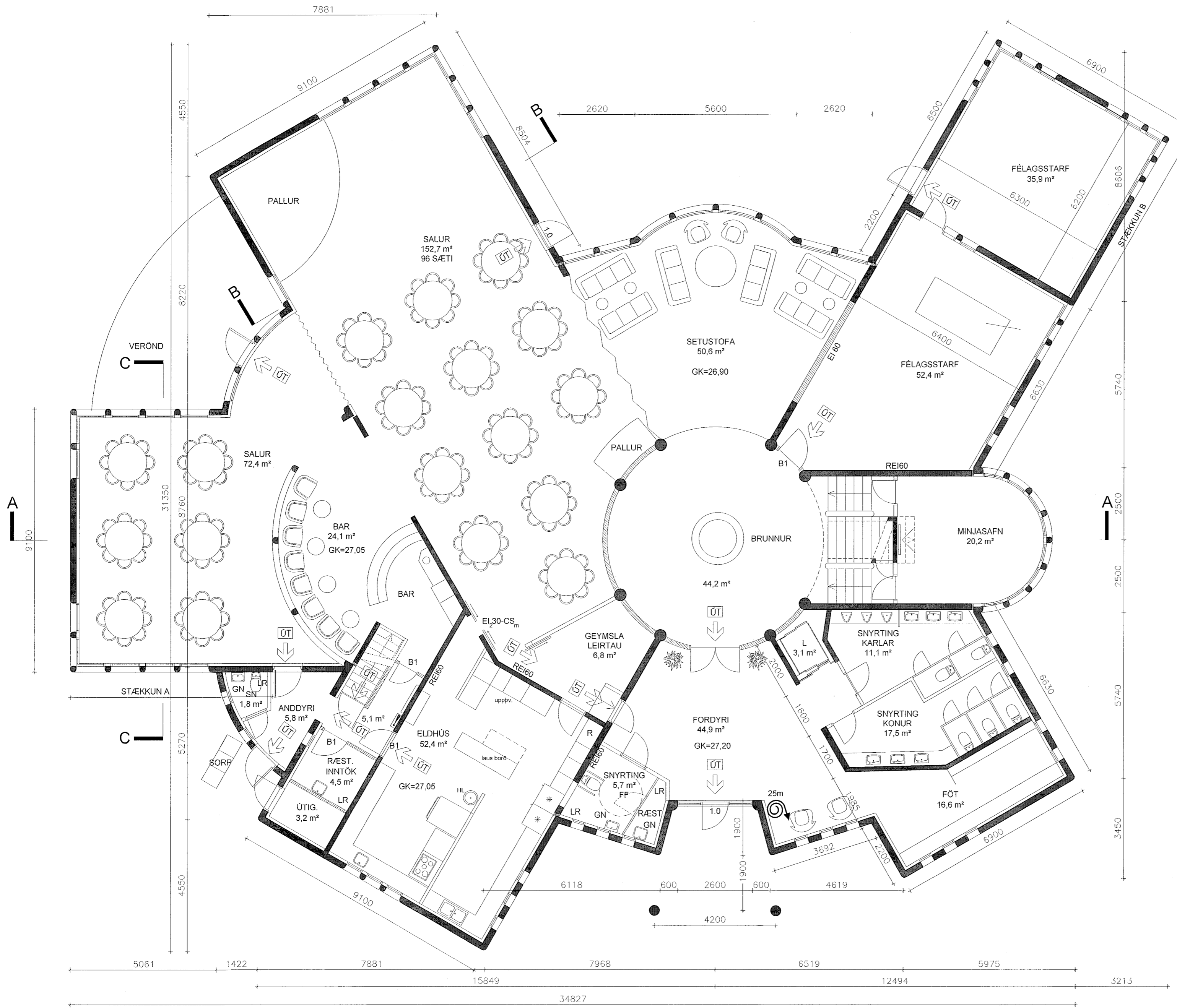
1 Grunnmynd 1. hæð 1 : 100
